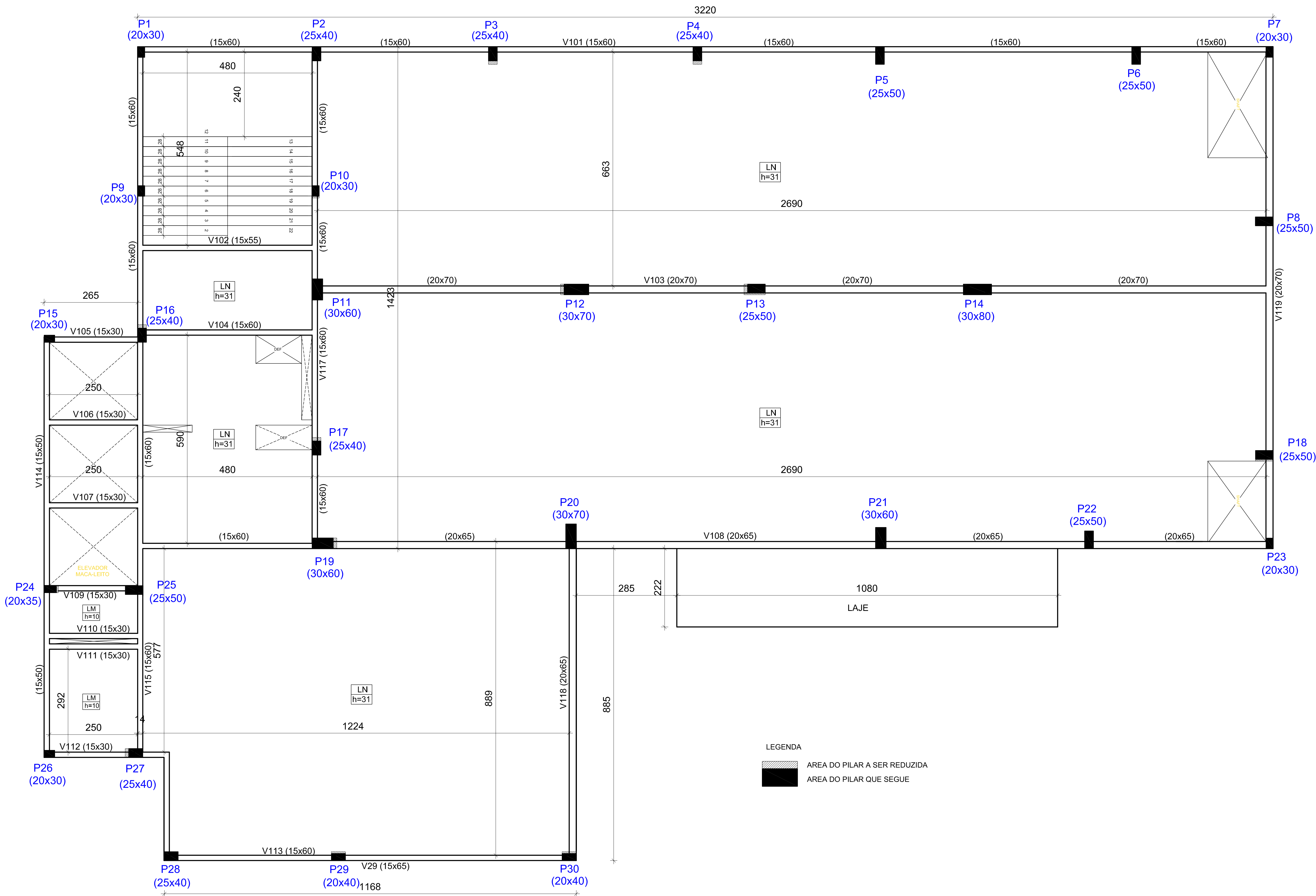
Planta de Fôrmas - 2º Pavimento Escala 1:50
